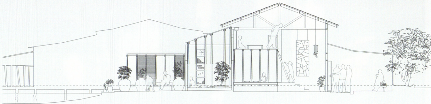
SECCIÓN LONGITUDINAL Y PLANTA BAJA LONGITUDINAL SECTION AND GROUND FLOOR
